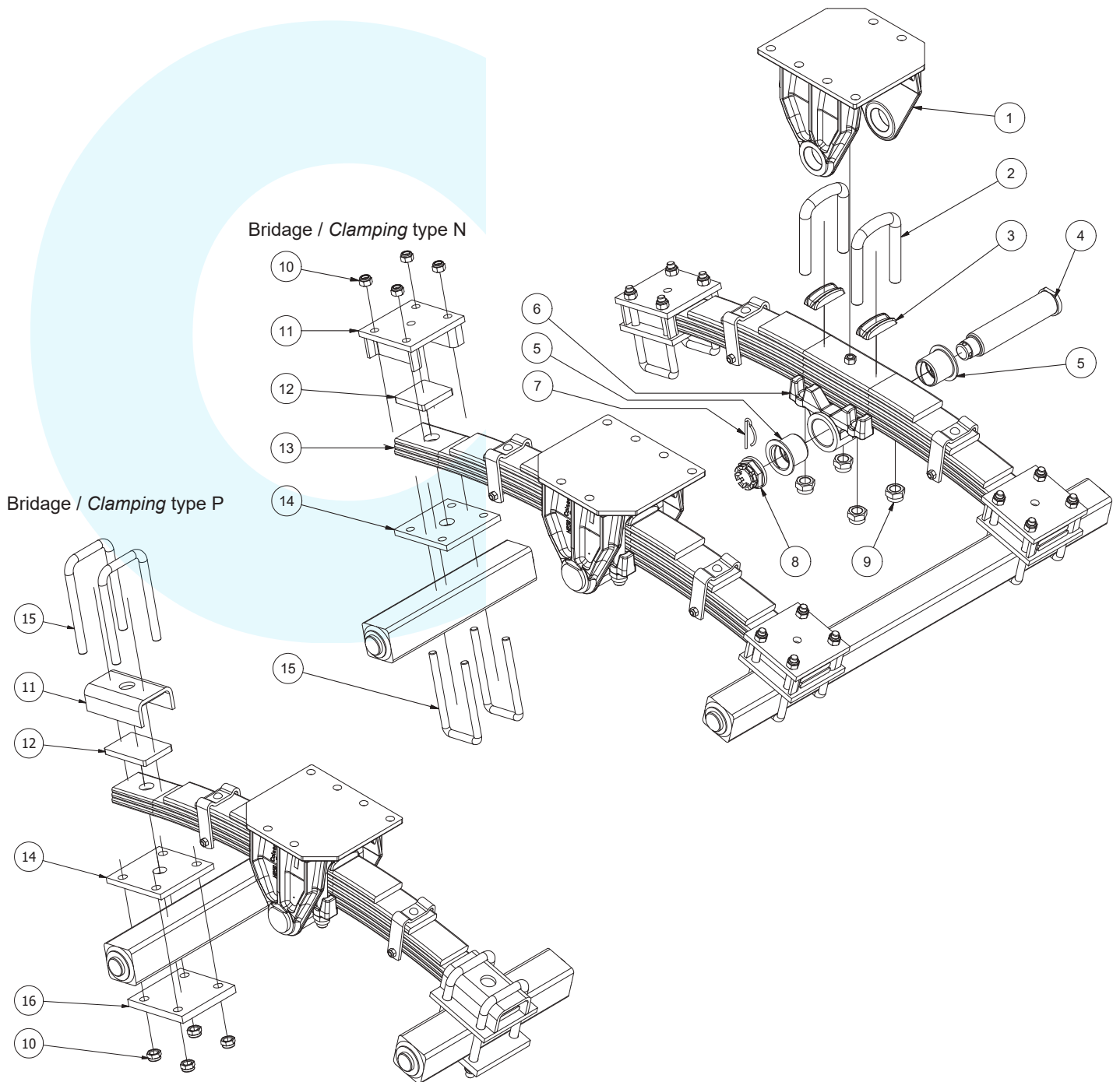
Vue éclatée (montage normal) Exploded View (normal mounting)
