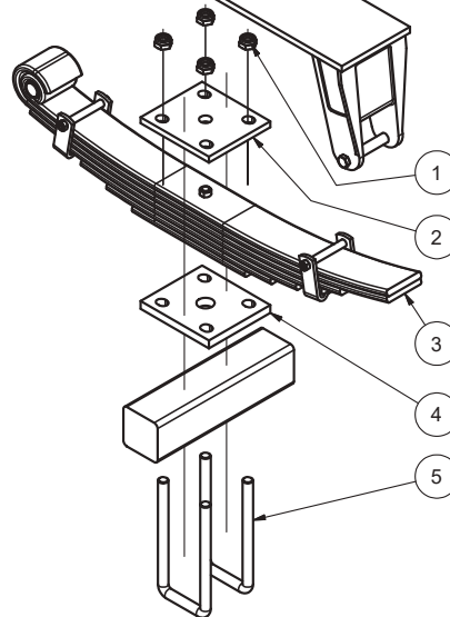
Bridage pour corps plein Clamping for full square
