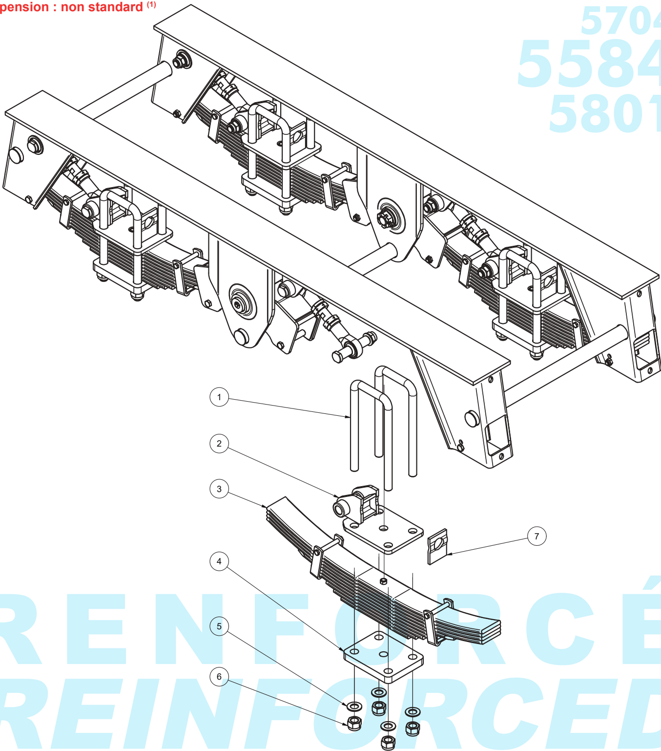
Vues éclatées montage surbaissé (suspension type tandem) / Exploded Views, underslung mounting (suspension type tandem)
