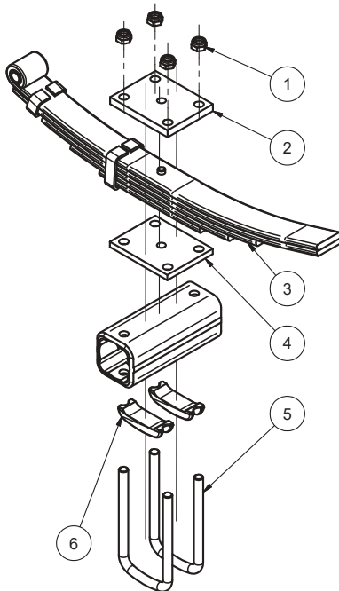
Bridage pour corps carré tubulaire Clamping for tubular square body
