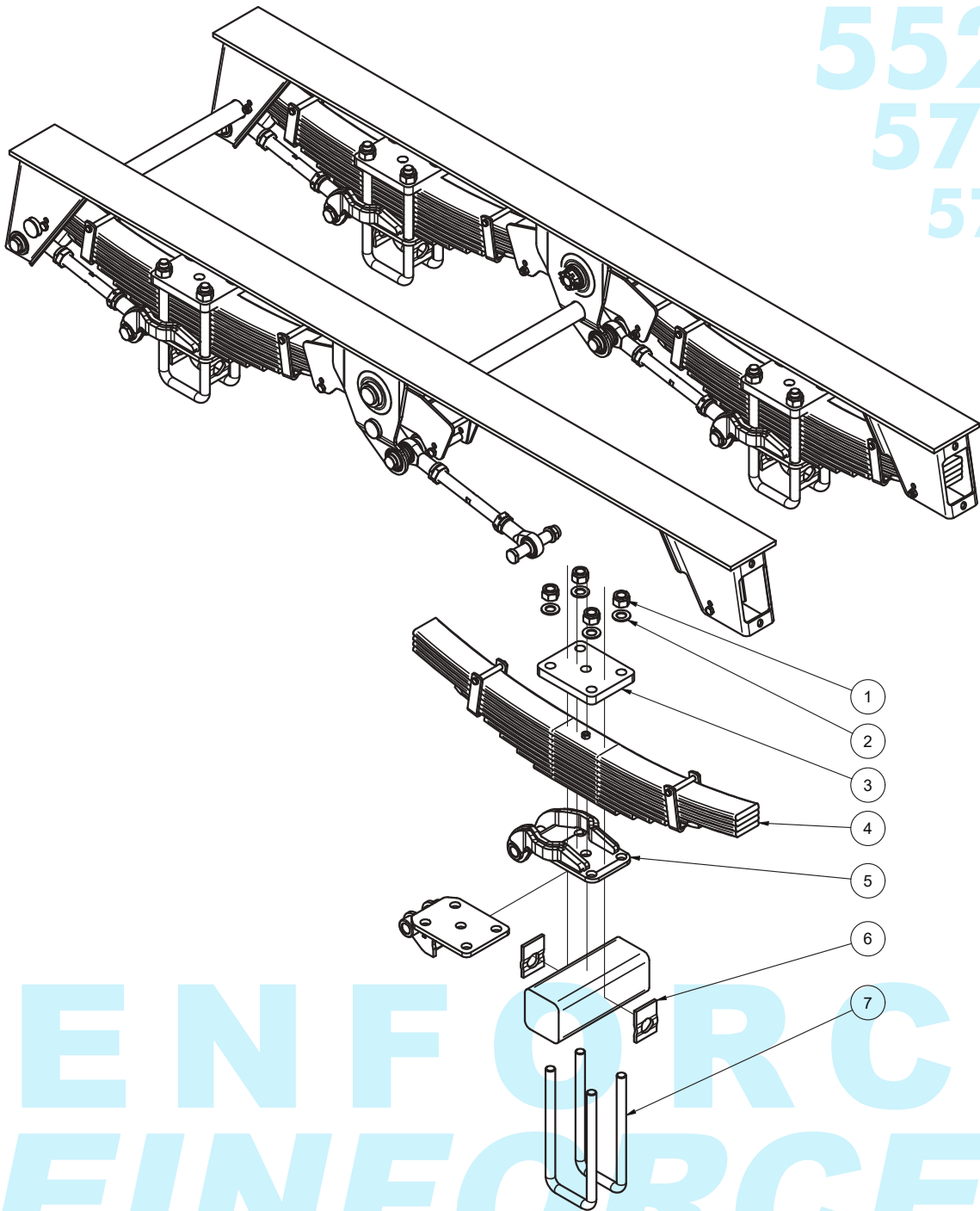
Vues éclatées montage normal (suspension type tandem) / Exploded Views, normal mounting (suspension type tandem)
