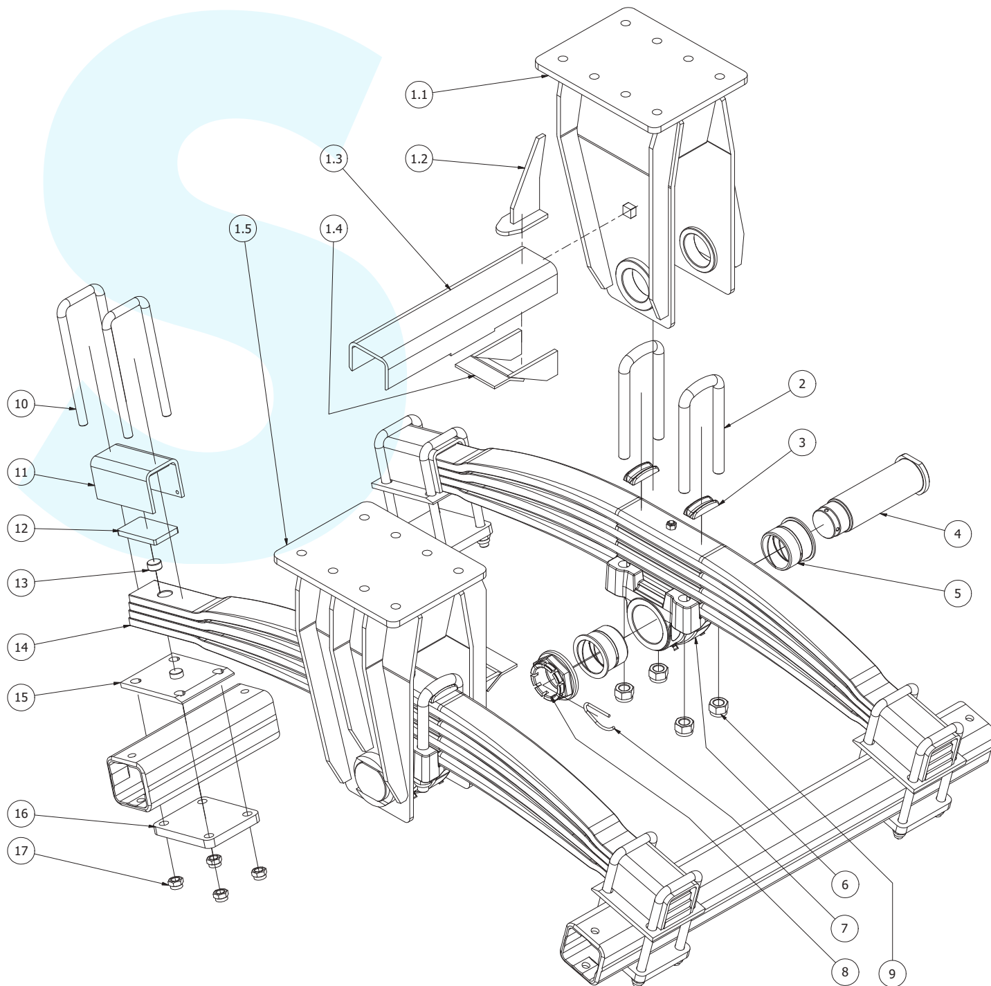
Vue éclatée (montage normal) Exploded View (normal mounting)
