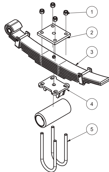
Bridage pour corps rond tubulaire Clamping for tubular round body
